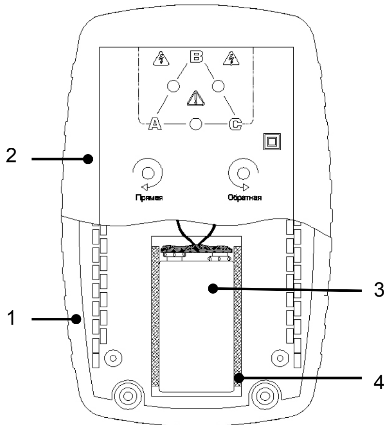
Рисунок 4.2 – Расположение батареи в указателе
